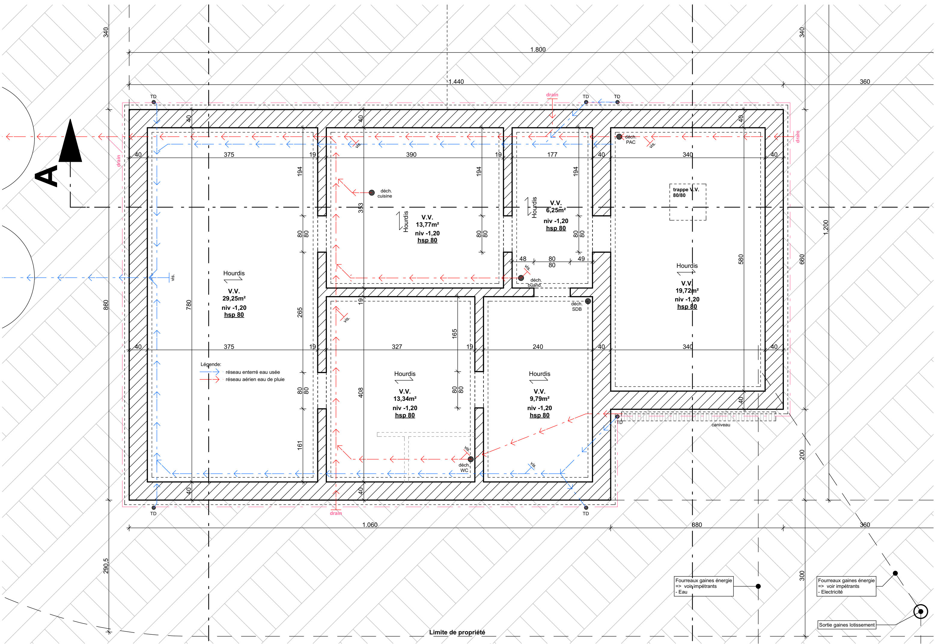
Plan V.V. 1/100
