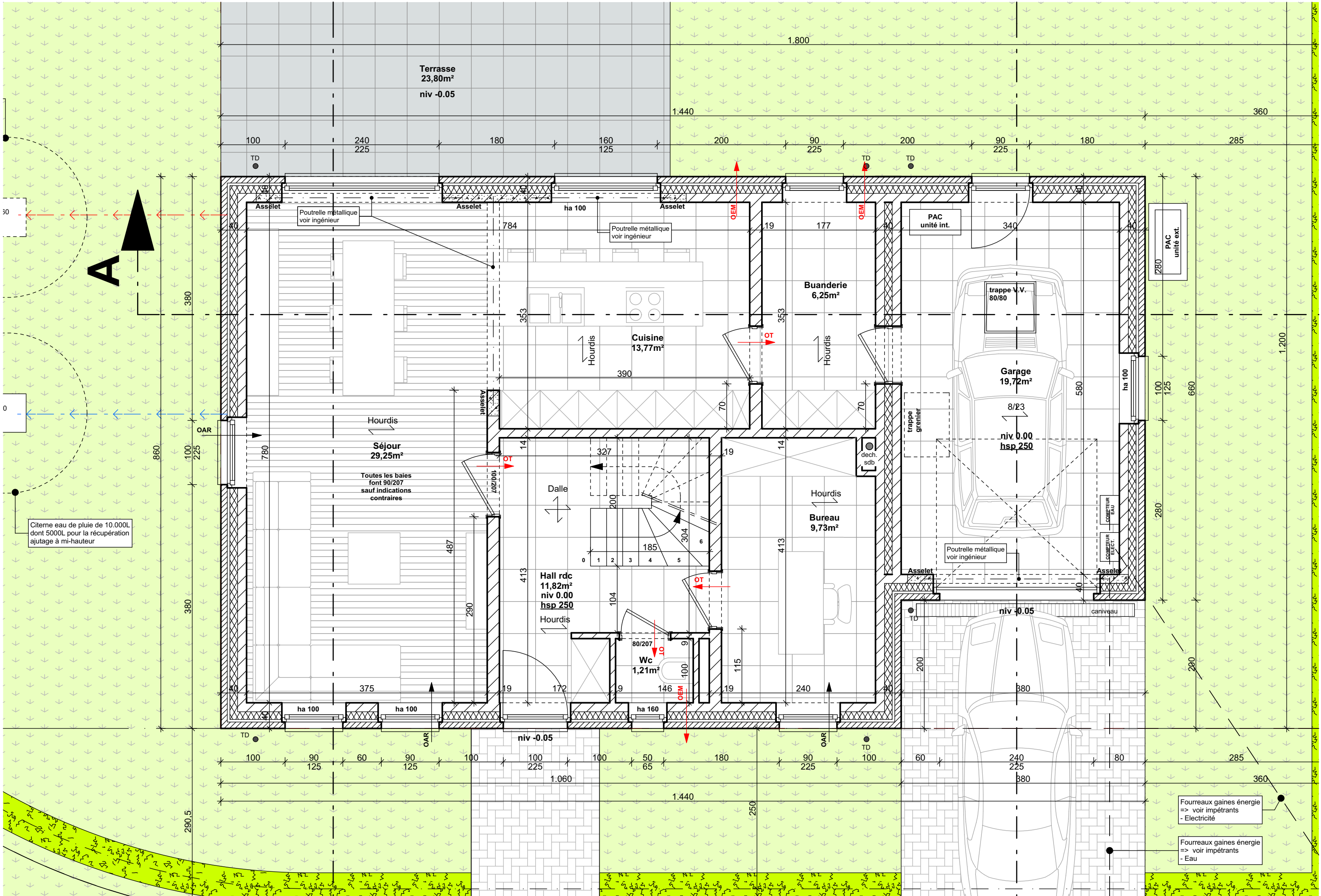
Plan rez-de-chaussée 1/50
