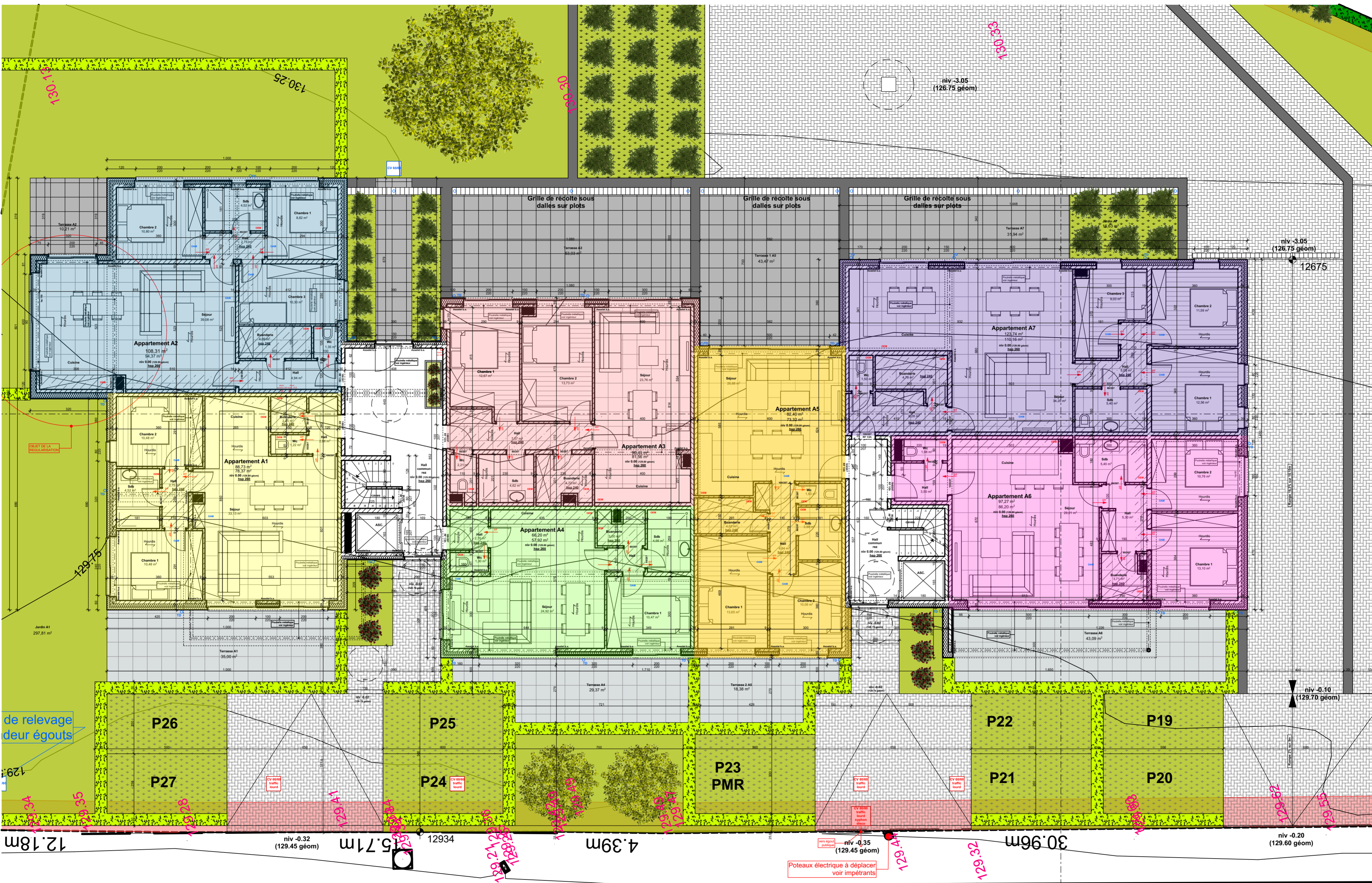
Plan rez-de-chaussée 1/100
