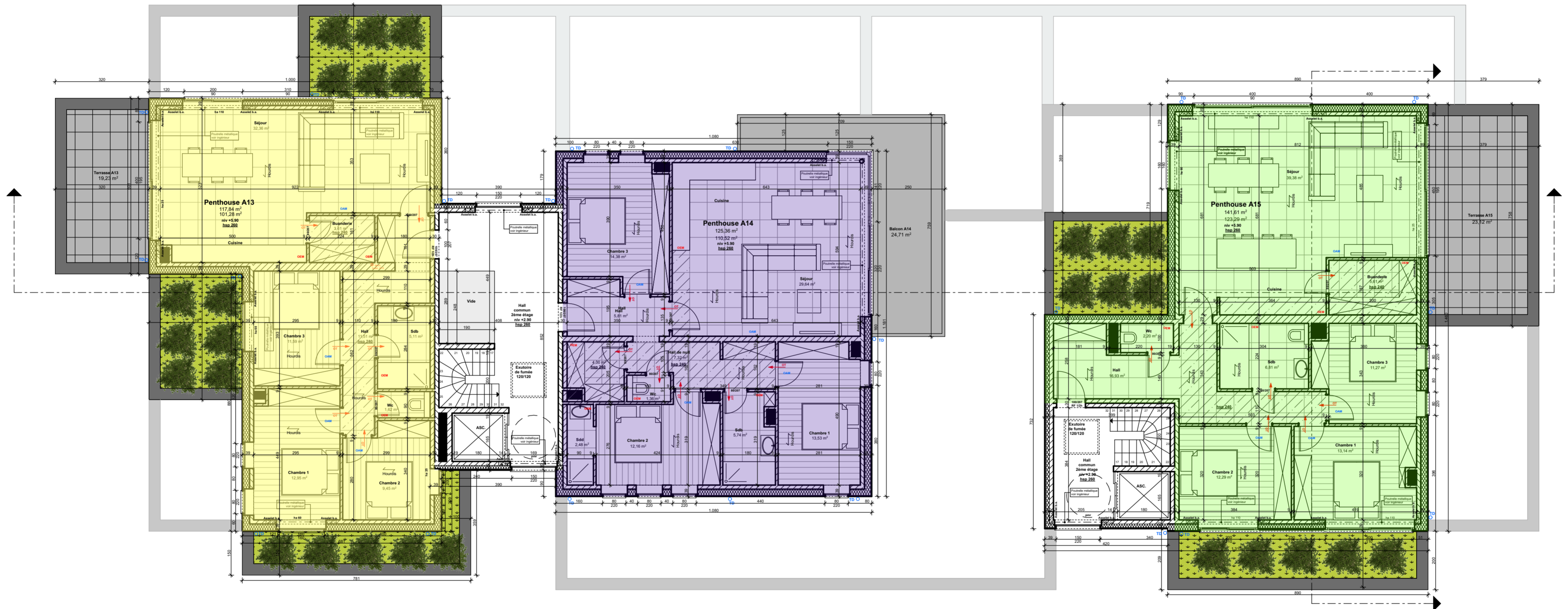
Plan 2ème étage 1/100
